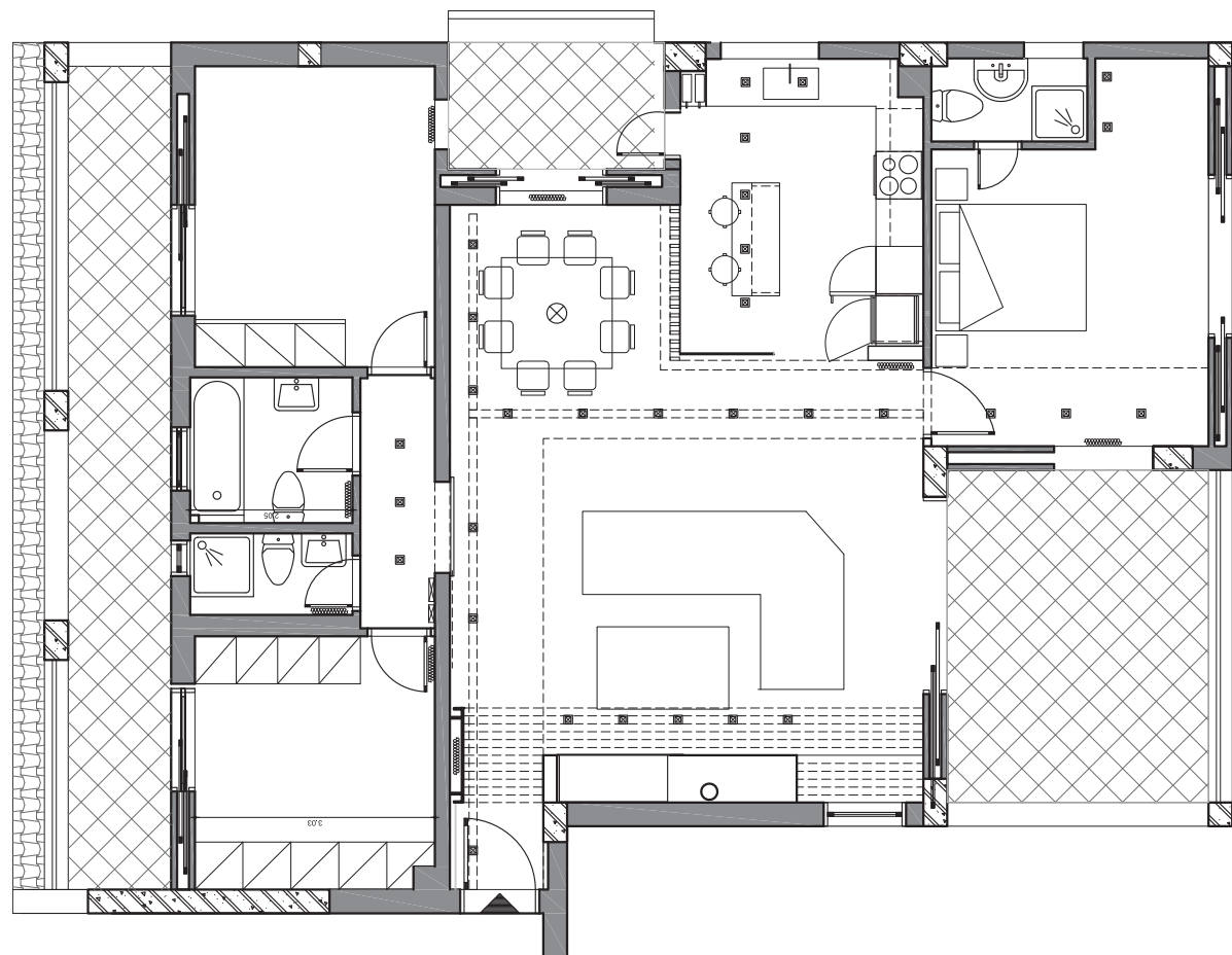
ΚΑΤΟΨΗ ΔΙΑΜΕΡΙΣΜΑΤΟΣ
