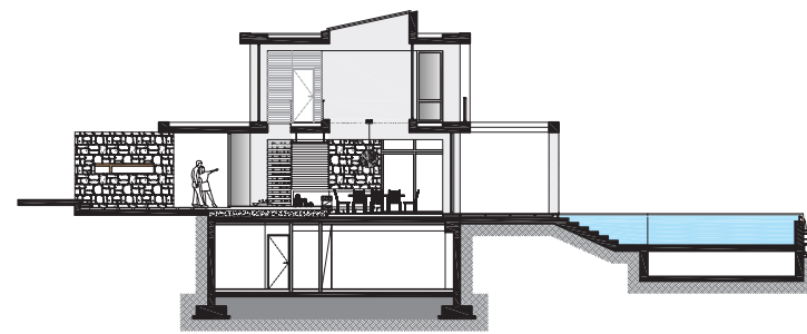
ΤΟΜΗ
