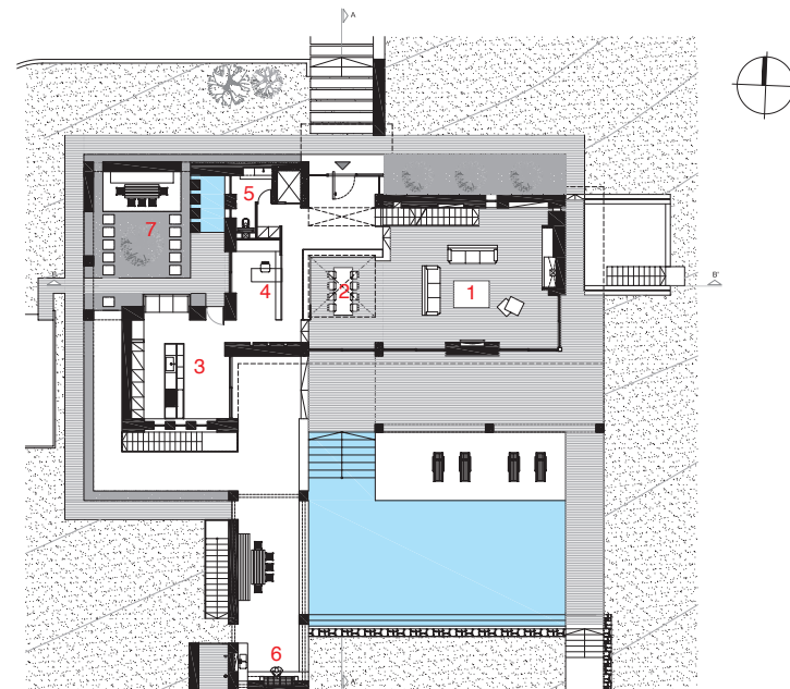
ΚΑΤΩΦΗ ΙΣΟΓΕΙΟΥ
